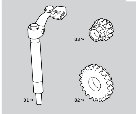
TIGE COMMANDE EMBRAYAGE PUSH ROD
