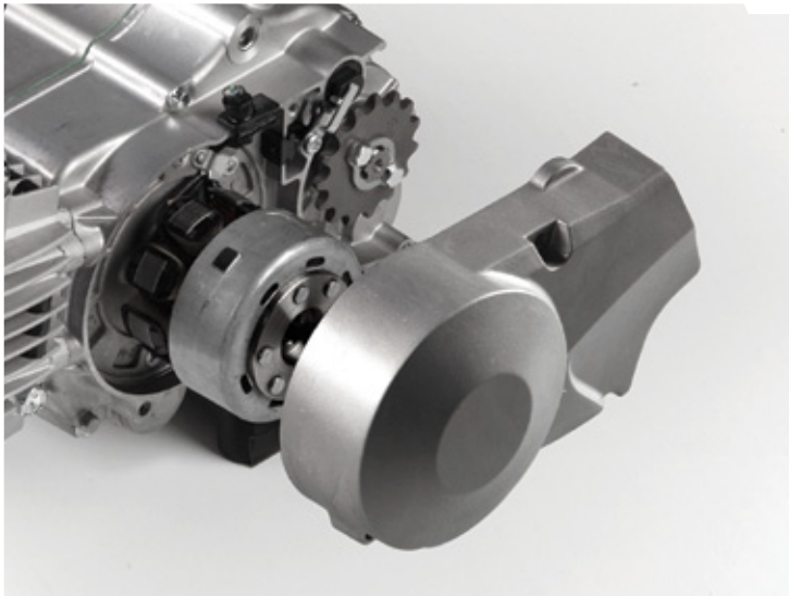
ALLUMAGE MAGNETO
