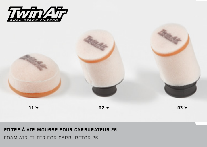
FILTRE À AIR MOUSSE POUR CARBURATEUR 26 FOAM AIR FILTER FOR CARBURETOR 26 01 → TA-158430 (POUR BOITE À AIR FACTORY/ FOR FACTORY AIR BOX) € 19 02 → TA-158432 (Ø 40mm POUR/ FOR MIKUNI® 26mm) 03 → TA-158431 (Ø 50mm POUR/ FOR KEIHIN® 28mm) € 24
