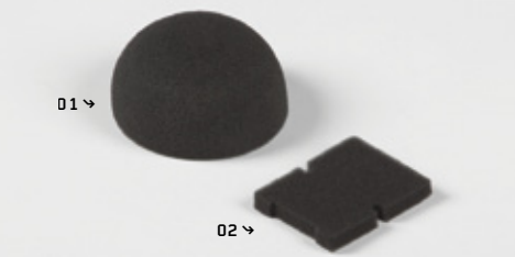
FILTRE À AIR EN MOUSSE FOAM AIR FILTER 01 → YC110-08-011 (FACTORY 2012-13) € 10 02 → YC50-0802 (POUR/ FOR YCF 50A) € 5
